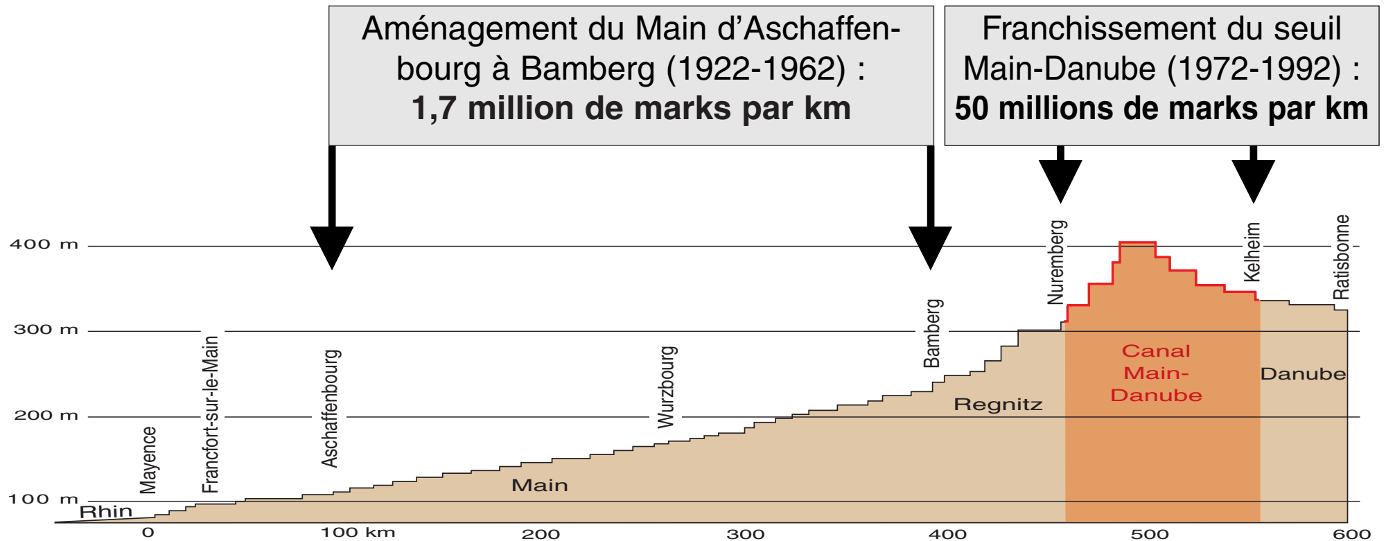
Liaison Rhin-Main-Danube : profil Mayence-Ratisbonne
